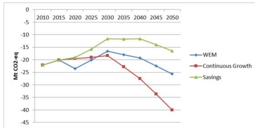
Nieluskenaariot
