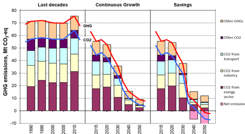
Kasvihuonekaasupäästöskenaariot
